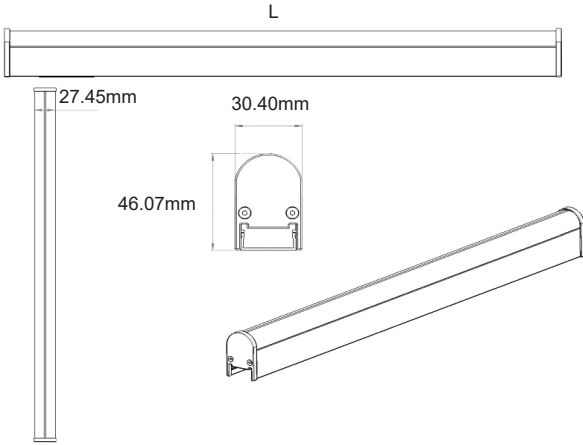
Profil Ölçüleri
